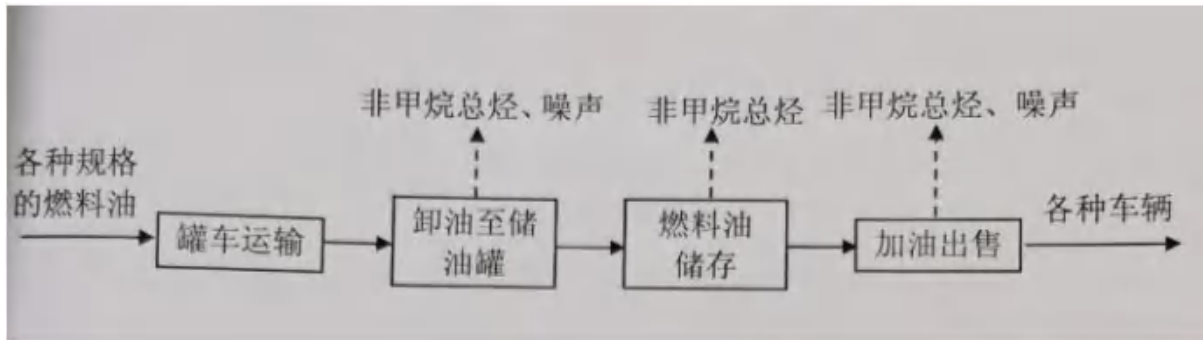
图 4.6-2 加油站工艺流程图
