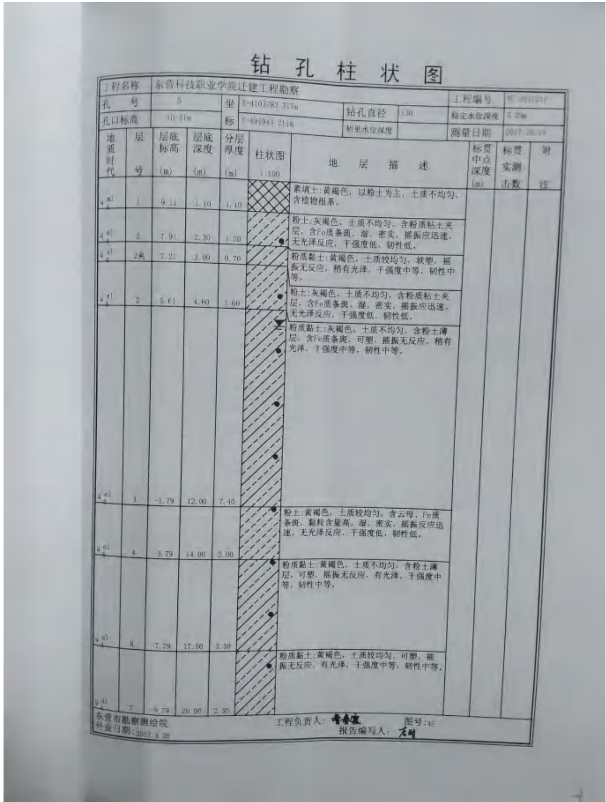
图 3.2-6 工程地质勘察柱状图（参考东营科技职业学院工程地质勘察报告）
