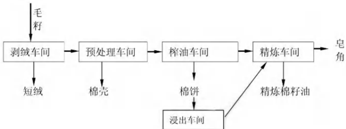
图 4.6-3 棉籽加工生产工艺流程图
