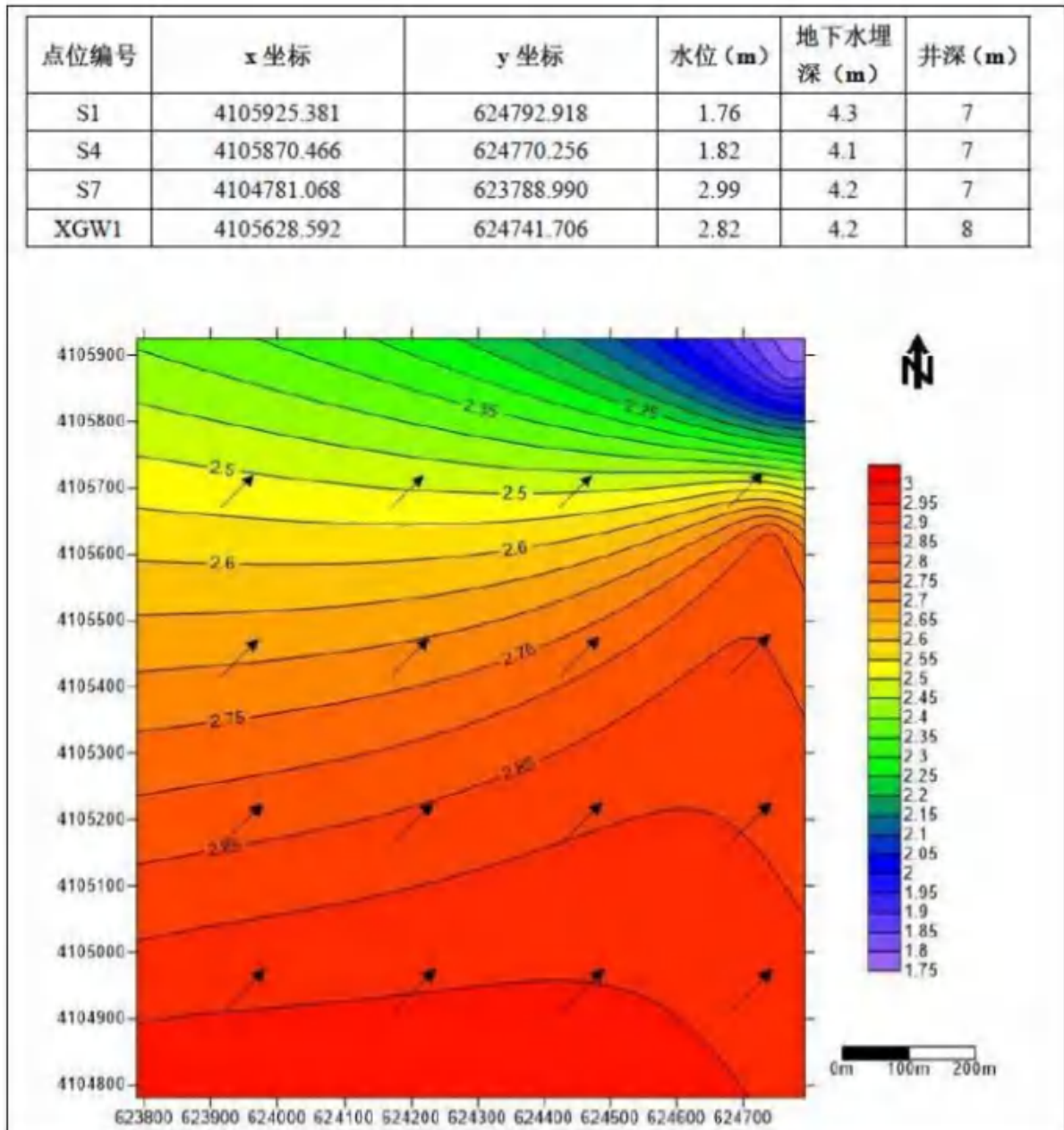
图 3.2-7 地下水流场图
